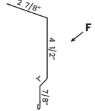
⑧ 29 Ga. Universal Sidewall TLUS8 10'2"
