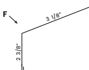
⑳ 29 Ga. Gutter Apron TLGA29 10'2"
