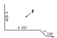
⑧ 29 Ga. Universal Sidewall TLUS8 10'2"
