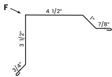
⑤ 29 Ga. Drip Cap TLDC9 10'2"
