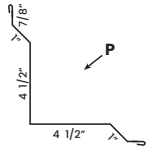
⑳ 29 Ga. Gutter Apron TLGA29 10'2"
